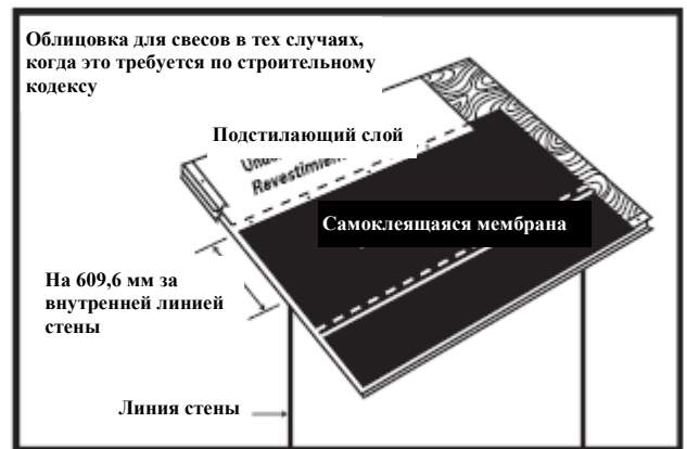
Рис. 2 Стандартный уклон ската для подстилающего слоя
